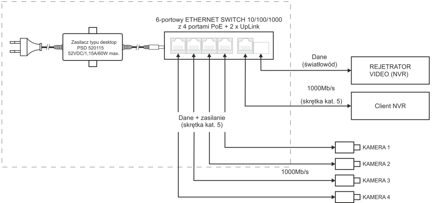
Rys. 1. Schemat blokowy.
